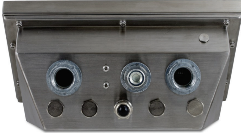
Figura 2-1: Centros de tubería eléctrica (conduit hub), caja para ambientes adversos
