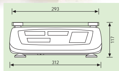
Mini-Tiger Dimensiones en mm
