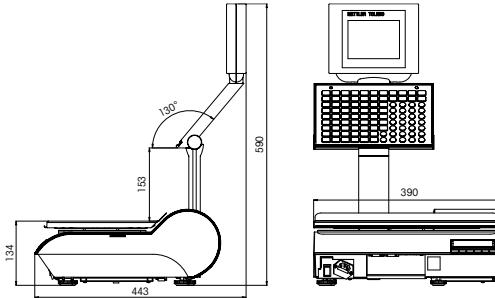
Wymiary bPro-U2
