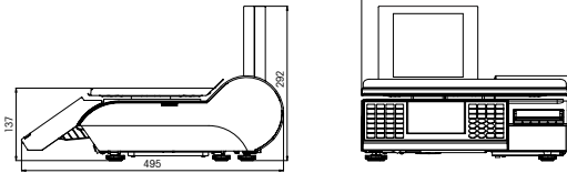
Wymiary bPro-C2
