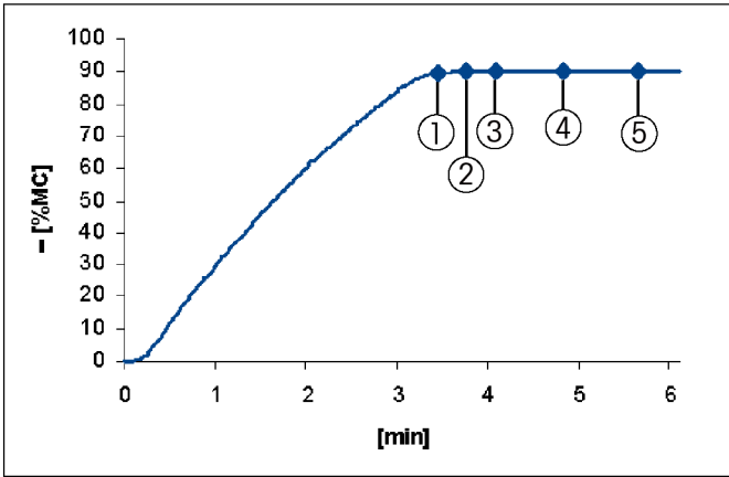
图B 用2.5克90%(重量百分比)氯酸钾溶液进行的一个试验性测量的干燥分布图(标准干燥，160℃)。图中示出了固定关机模式1至5。一旦达到关机模式2，则结果仅稍有变化。为了获得目标值(90%)，AutoMet推荐关机模式3。
