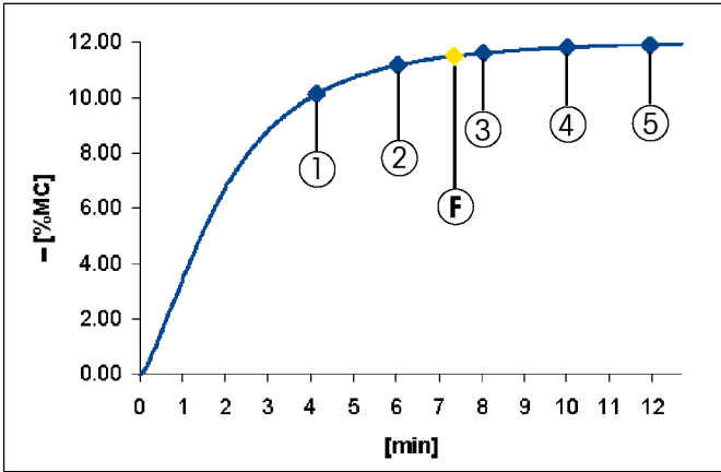
图A 用2.5克细粉进行的一个试验性测量的干燥分布图(标准干燥，100℃)。图中示出了固定关机模式1至5，以及用AutoMet确定的关机模式F(1mg/35秒)，用关机模式F获得精确目标值(11.48%)。
