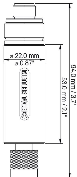
Schéma technique du transmetteur M80 SM
